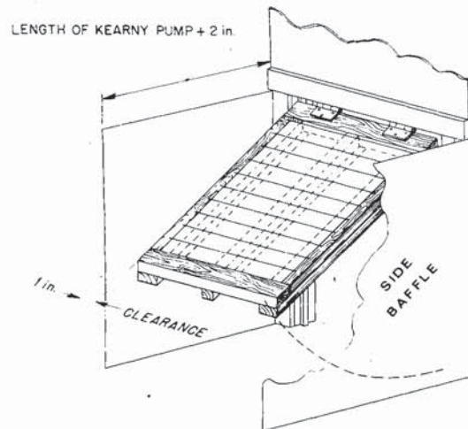
Fig. 25. Side baffles.
