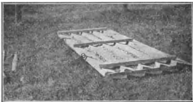
FIG. 1. PLANK DRAG
